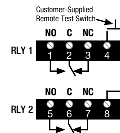
Relay Wiring APD 1420
